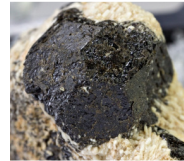
Kimzeyite - Arkansas
